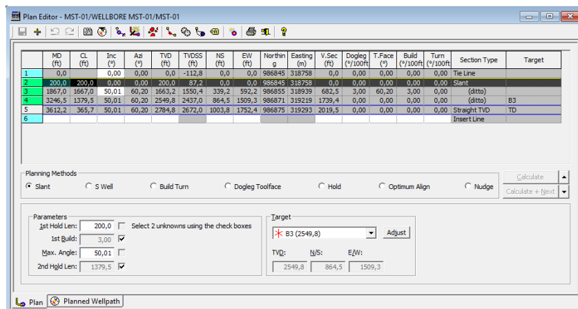
Gambar 7. Perencanaan Vertikal Build Section
