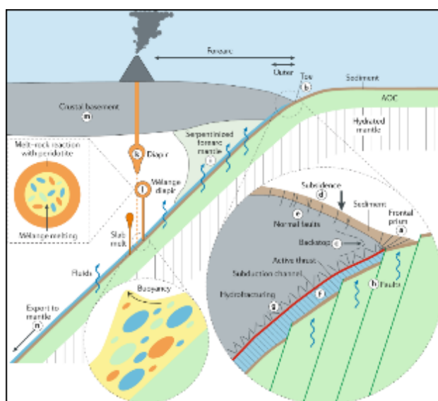
Gambar 1. Model konseptual pembentukan magma pada zona subduksi
