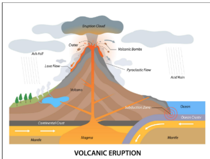
Gambar 4. Mekanisme erupsi vulkanik
