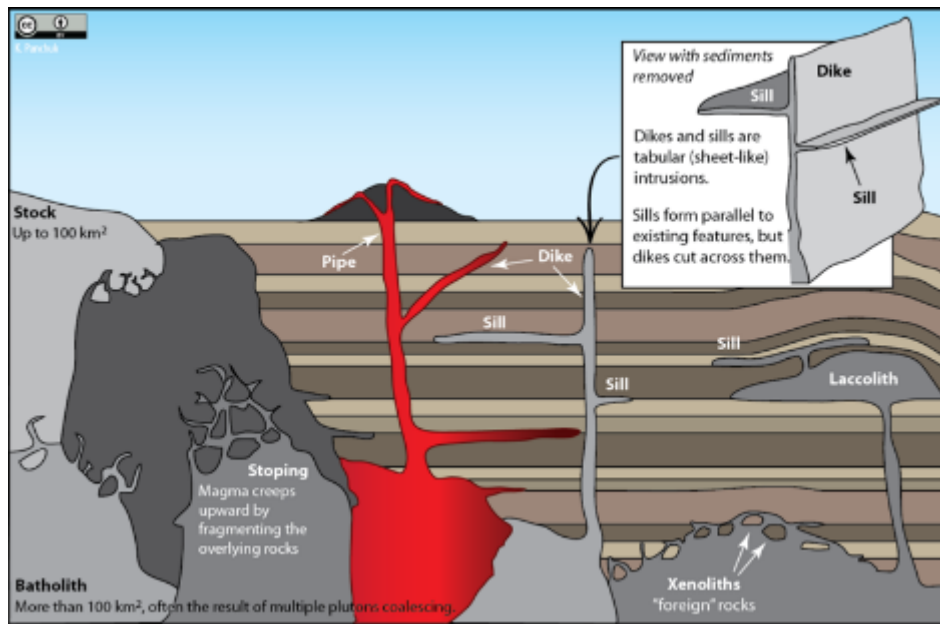
Gambar 3. Berbagai tipe intrusi magmatik
