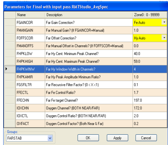
Gambar 10 Input Far Parameter untuk Log Average (Microsoft, 2007)
