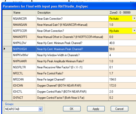
Gambar 9 Input Near Parameter untuk Log Average (Microsoft, 2007)
