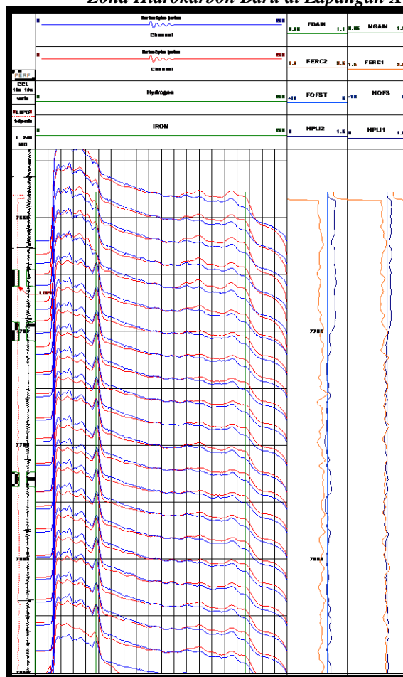
Gambar 6 Log untuk Gain Stabilization
