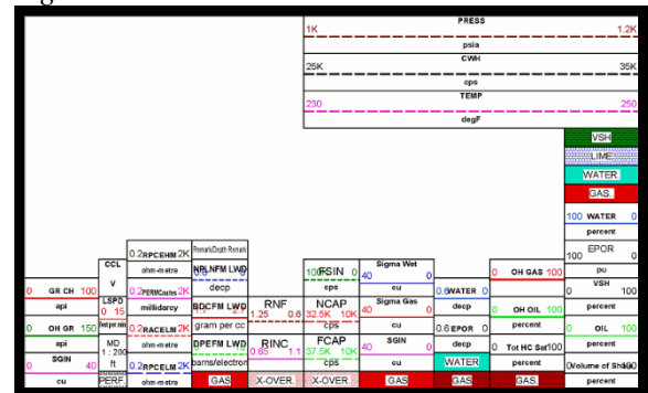
Gambar 13. Kepala Log dari Sigma Saturation
