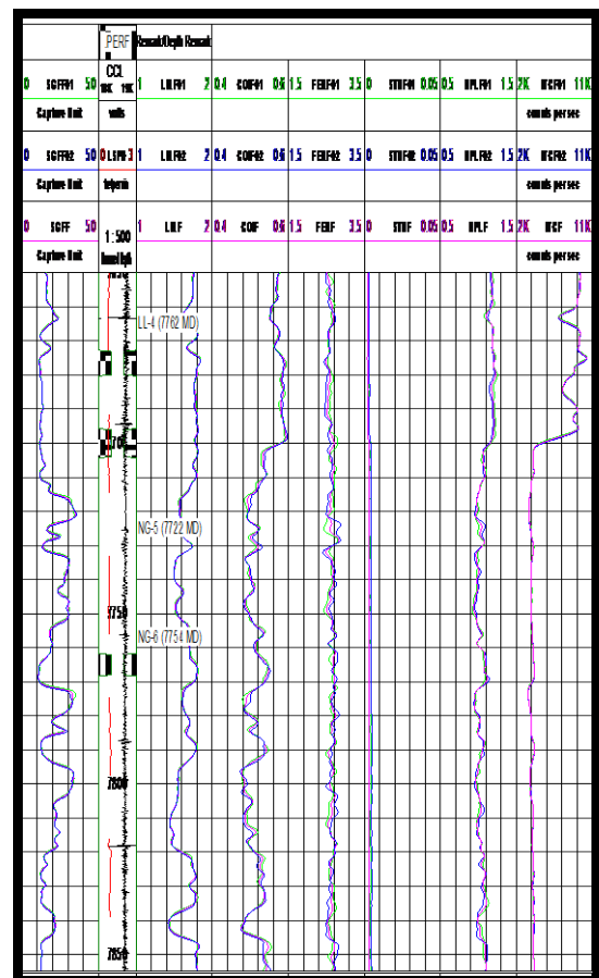
Gambar 11 Log Average untuk C/O3.
