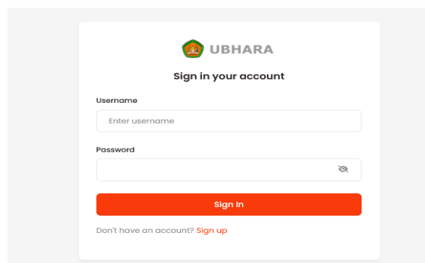
Gambar 6. Halaman Login
