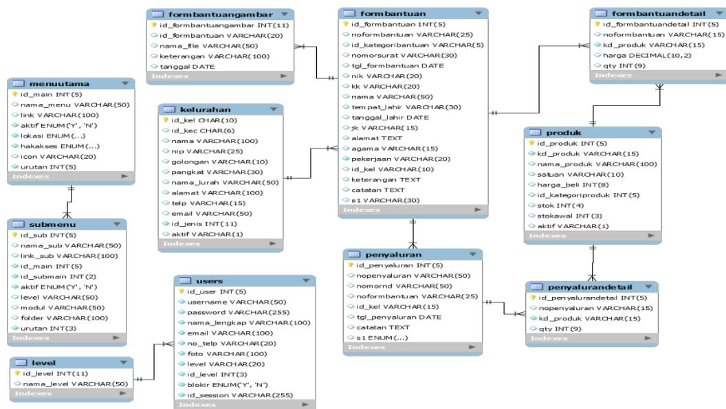
Gambar 3. EERD
